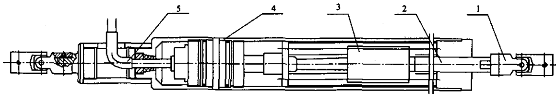
1—万向节；2—位移杆；3—敏感元件；4—密封壳体；5—引出电缆
