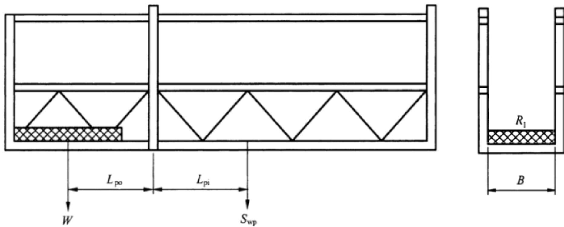
图 6 悬臂平台
