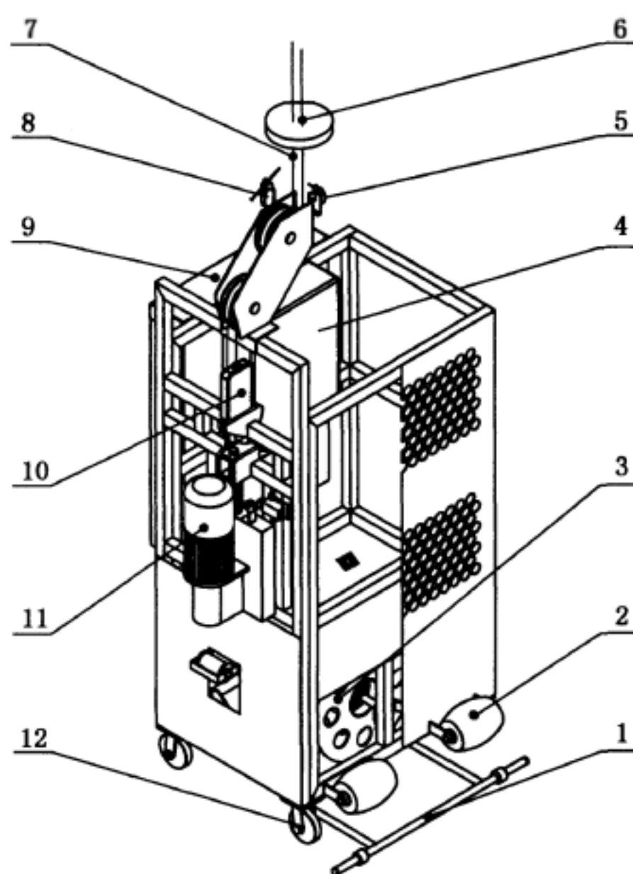
图2 双吊点平台
