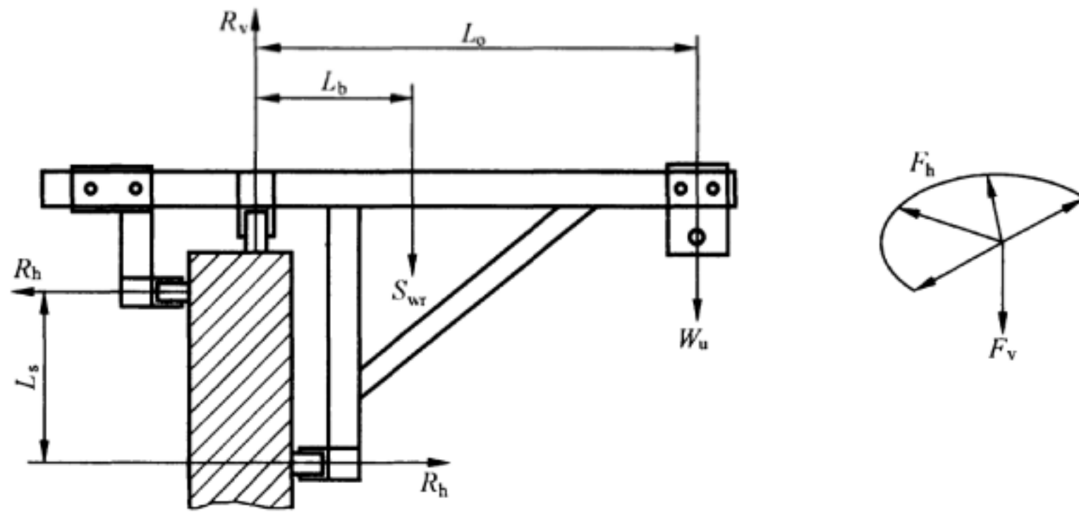
图 11 女儿墙卡钳
