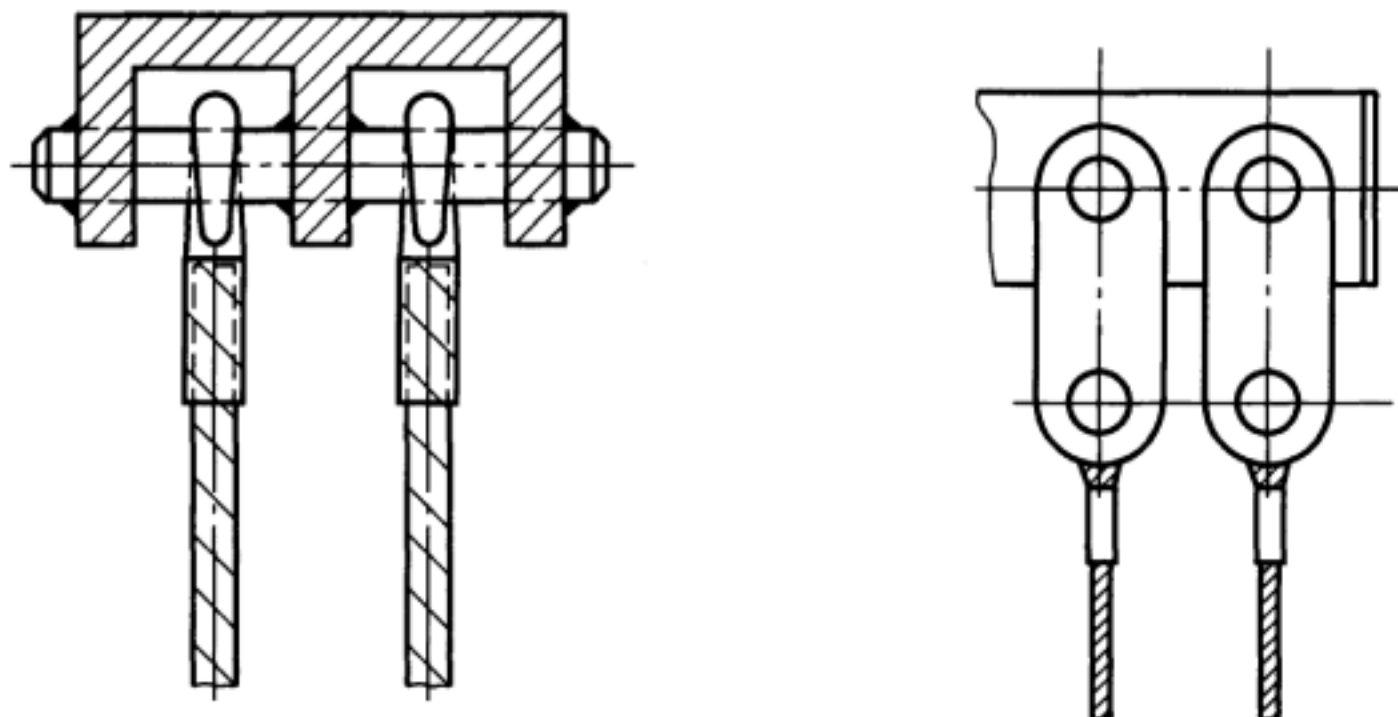
图 16 典型悬挂点示例
