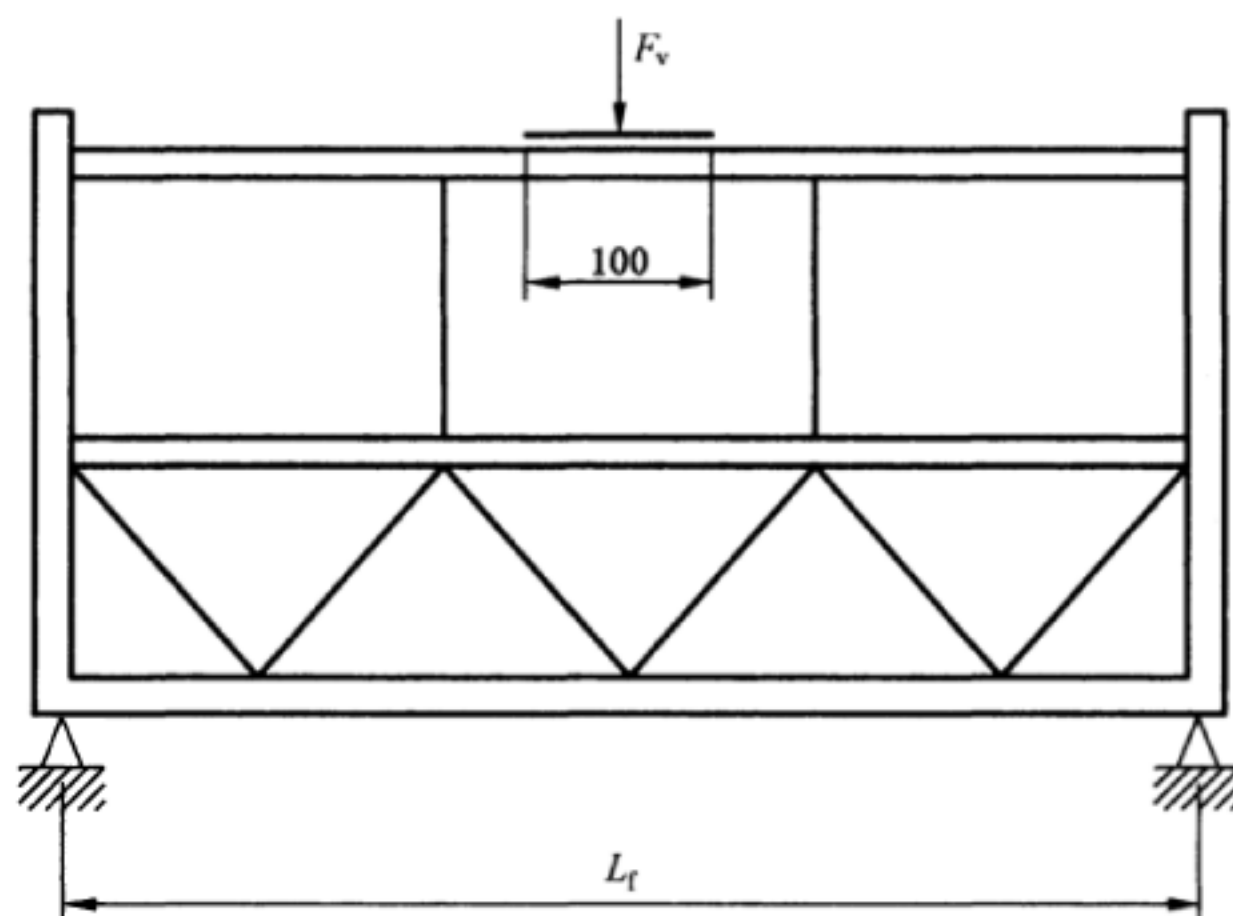
图 A.5 护栏上的垂直载荷
