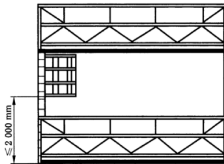
图 14 多层平台
