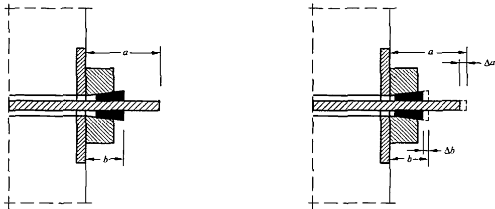
a) 锚固之前,预应力筋顶紧之后
