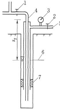
图 B.0.8-2 回水管上安设压力表示意图
