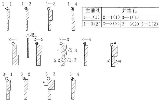
图 D03 深孔固结灌浆成果综合平、剖面图
