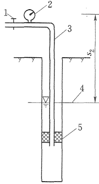
图 B.0.8-1 进水管上安设压力表示意图
