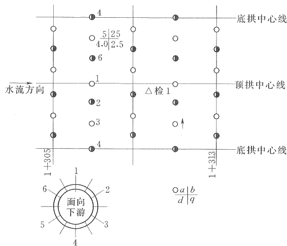
图 D04 隧洞固结灌浆成果展示图
