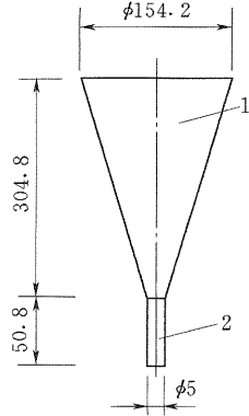
图 A.3.2 马氏漏斗黏度计示意图 (单位：mm)
