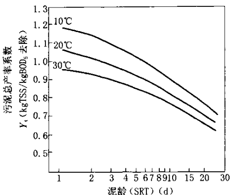
图3 无初次沉淀池时泥龄-污泥总产率系数曲线
