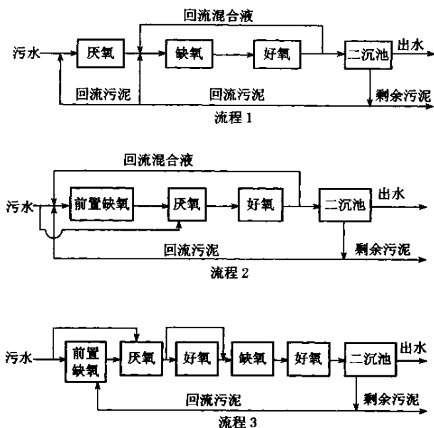
图 4 一些变形的工艺流程
