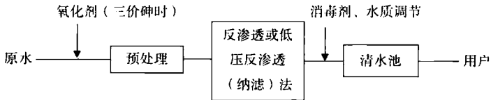
图 9.8.23 反渗透或低压反渗透(纳滤)法除砷工艺流程
