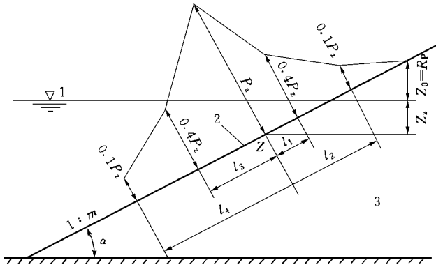
图A. 1.16 坝坡护面板上的波浪压力
