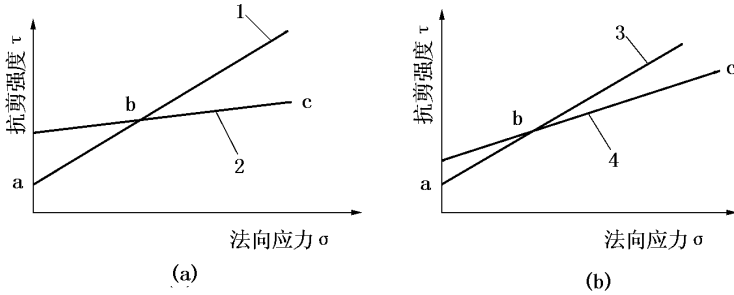
图D.1.3-1 弧度包线的组合
