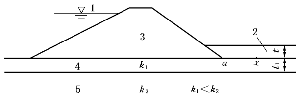
图8.2.4 坝基结构示意图
