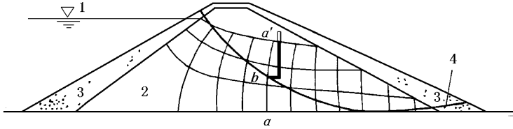
图C.0.3 稳定渗流流网示例
