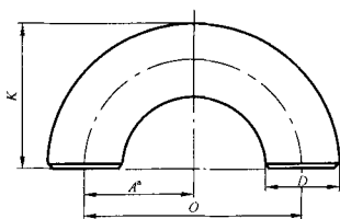
图 5 短半径 180°弯头
