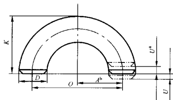
图 3 长半径 180°弯头
