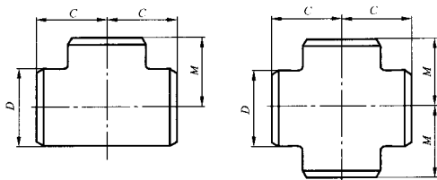
图 6 等径三通和四通
