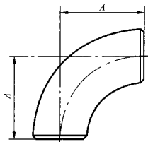
图 A.5 短半径弯头
