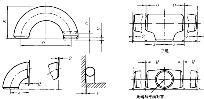
图 A.1 公差简图
