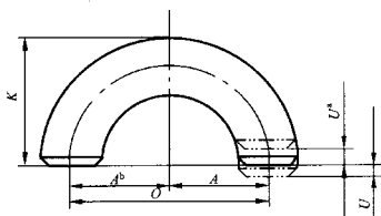
图 A.4 长半径 180°弯头
