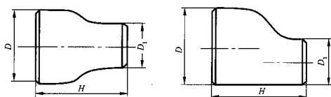
图 10 异径接头
