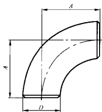
图 4 短半径弯头
