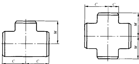
图 A.8 异径三通和四通
