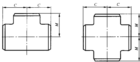
图 A.7 等径三通和四通
