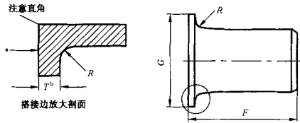
图 A.9 翻边短节 表 A.9 翻边短节尺寸
