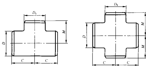
图 7 异径三通和四通
