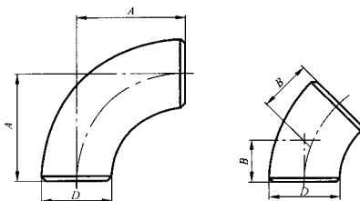
图 1 长半径弯头
