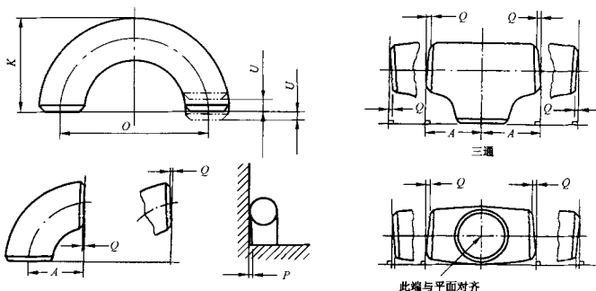
图 11 公差简图
